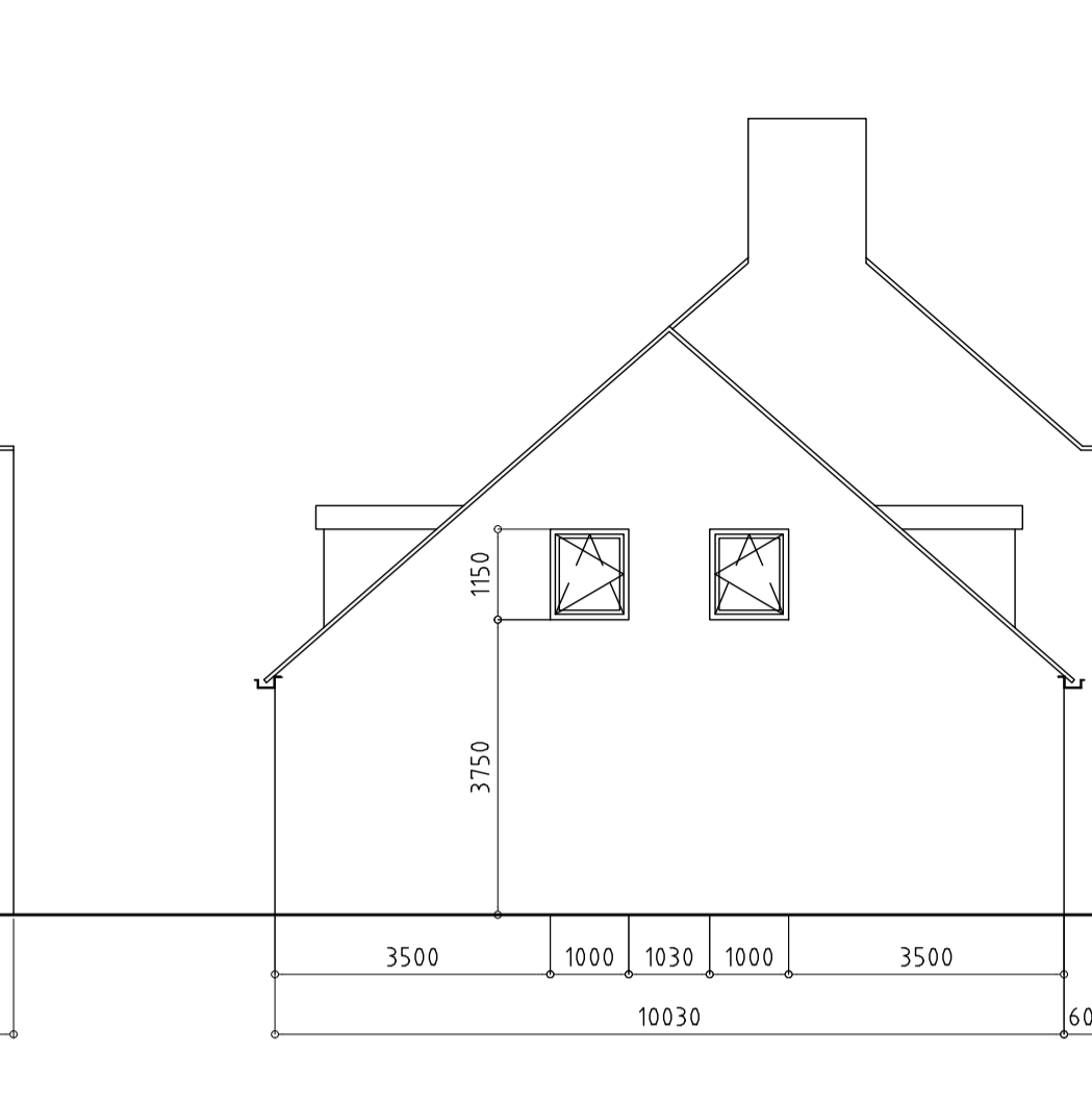
ZIJGEVEL NIEUW
