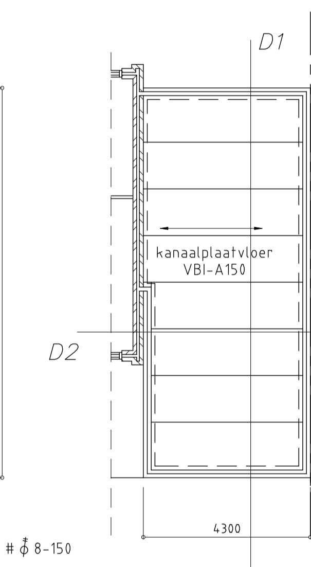
VLOER 1e VERD.
