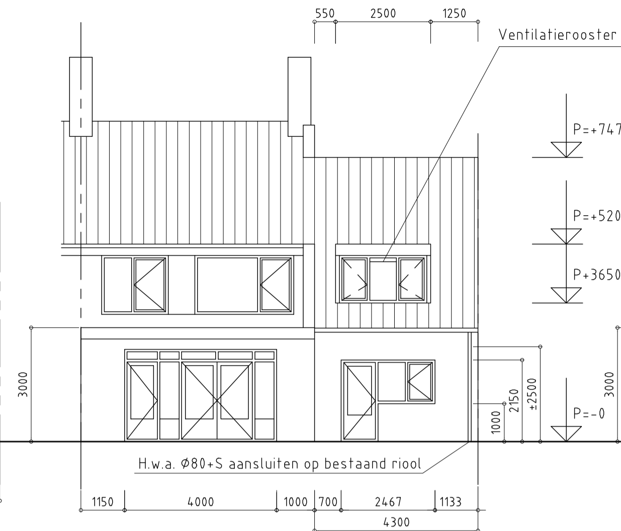
ACHTERGEVEL NIEUW
