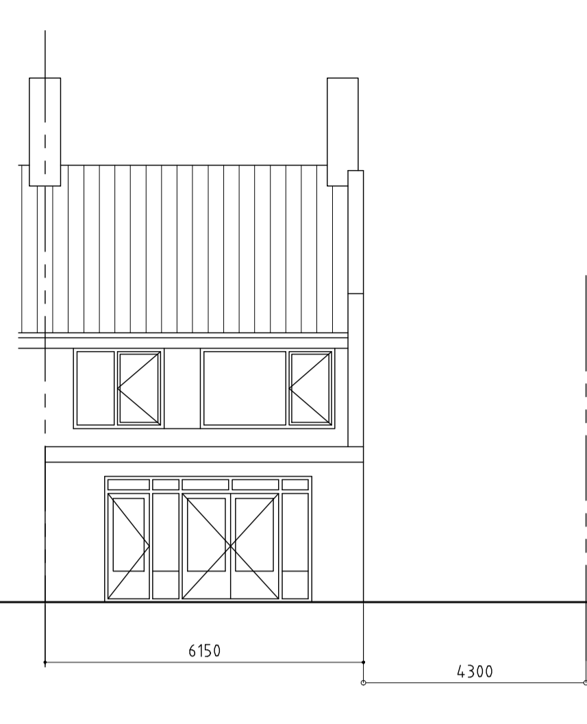
ACHTERGEVEL BESTAAND
