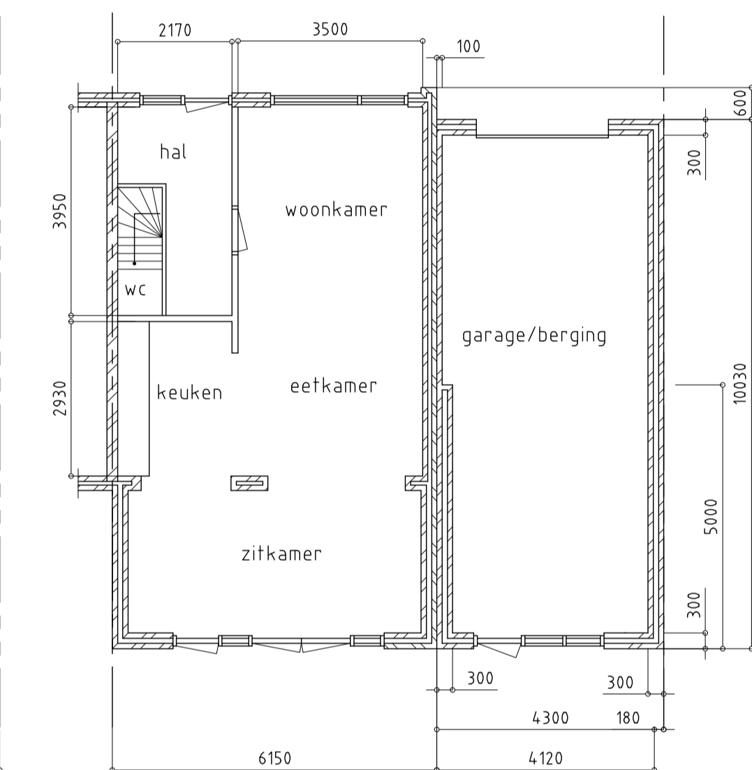
BEGANE GROND NIEUW
