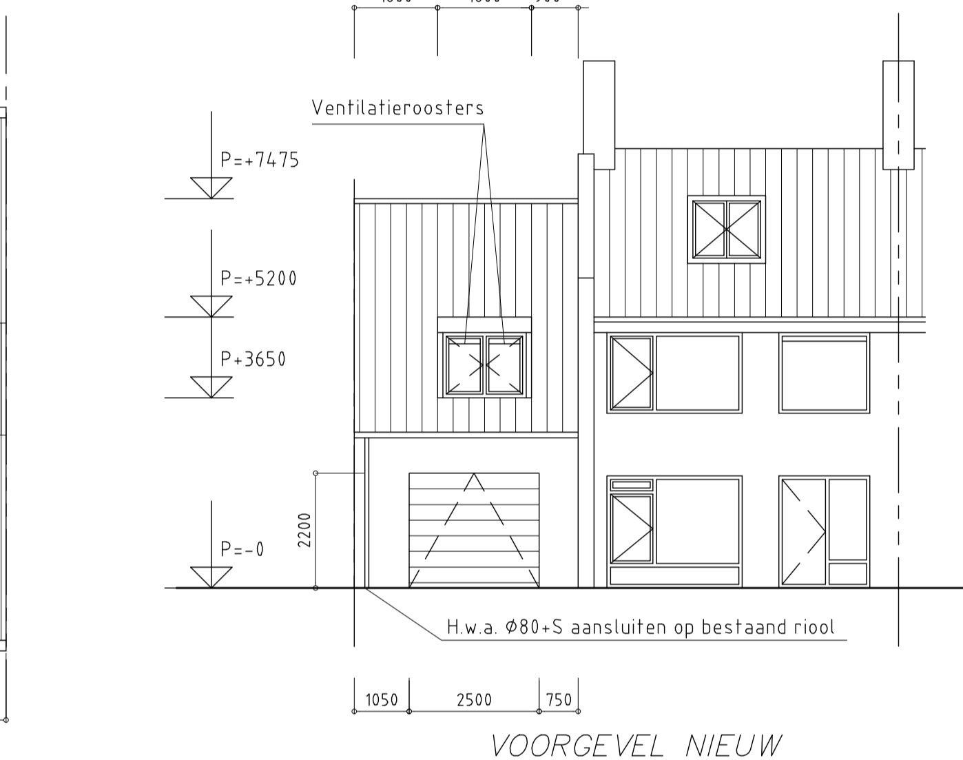
VOORGEVEL NIEUW
