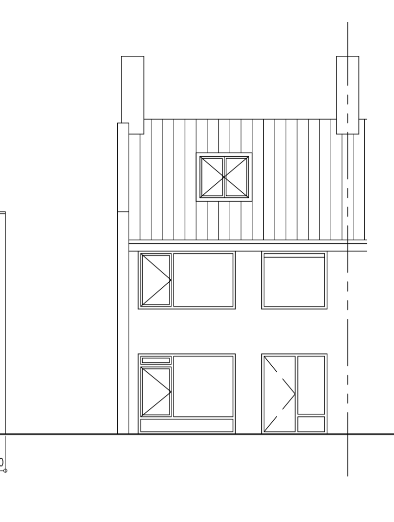
VOORGEVEL BESTAAND
