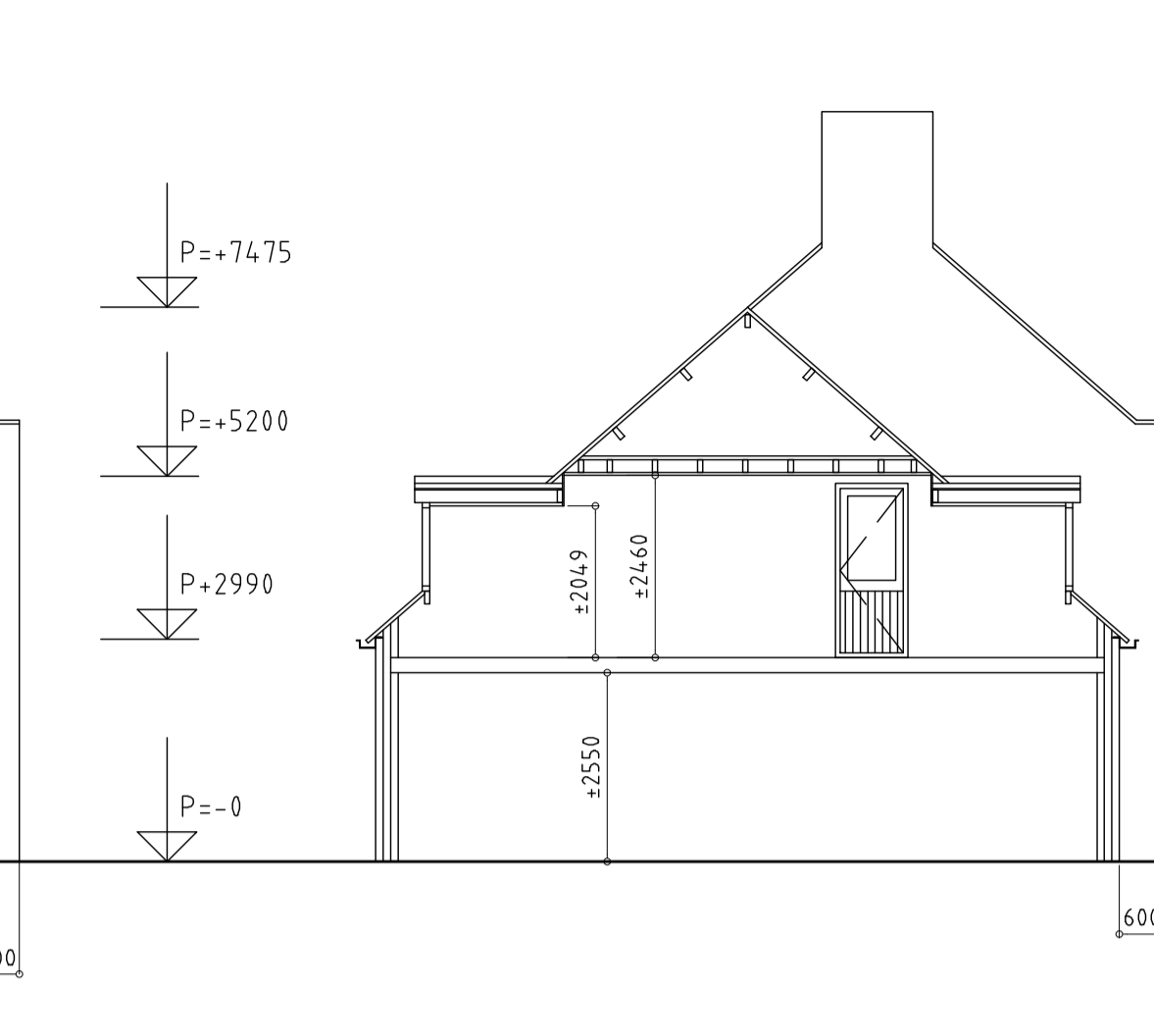
DOORSNEDE NIEUW
