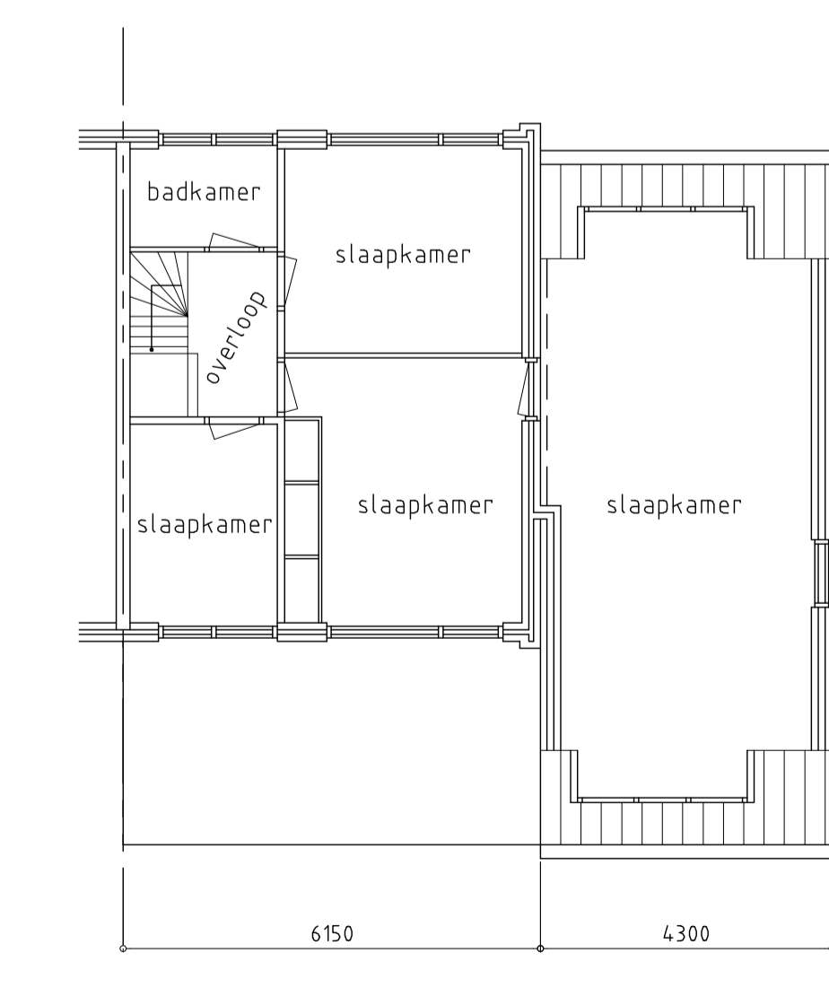
2e VERDIEPING NIEUW
