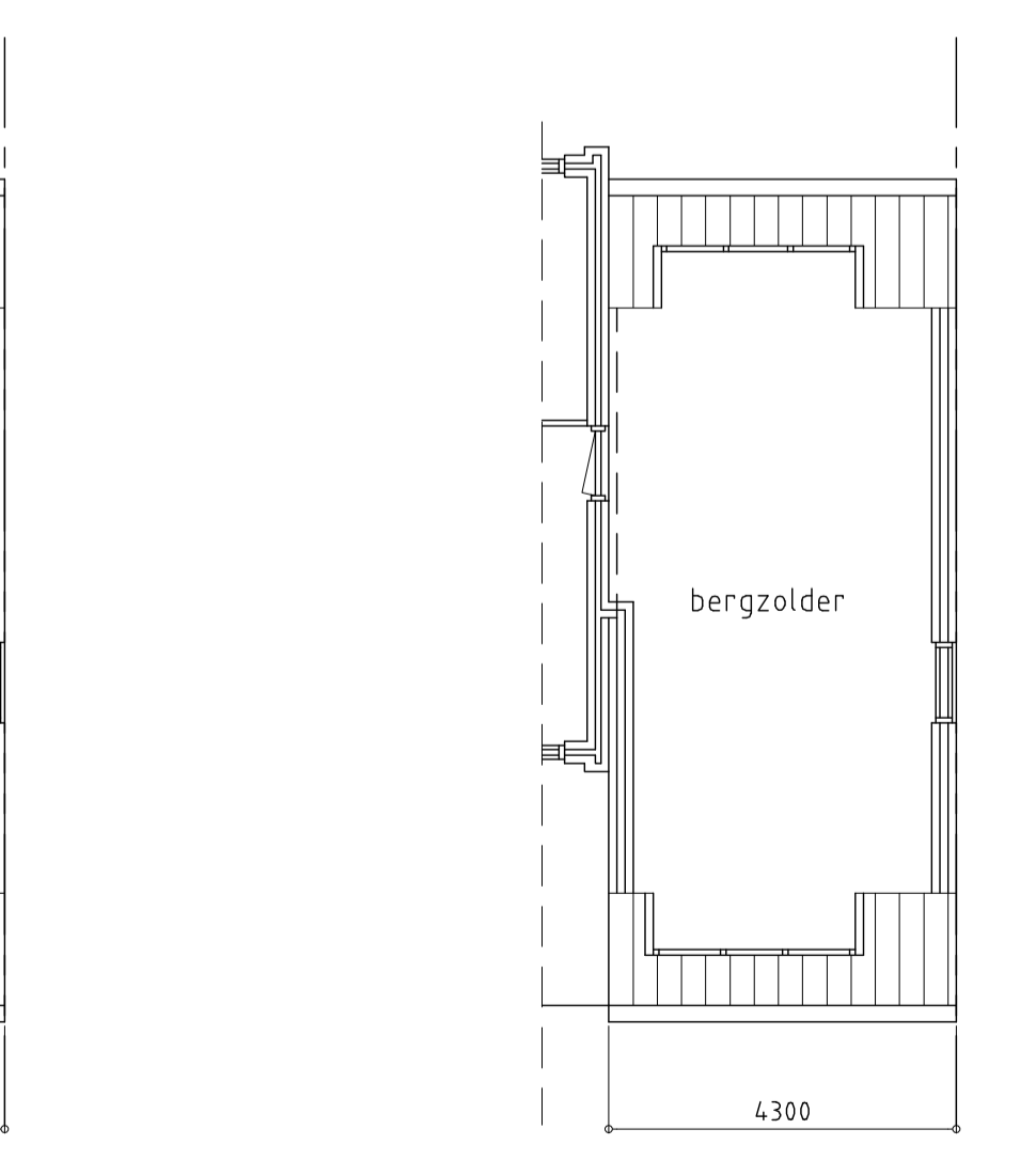
KAPPLAN
