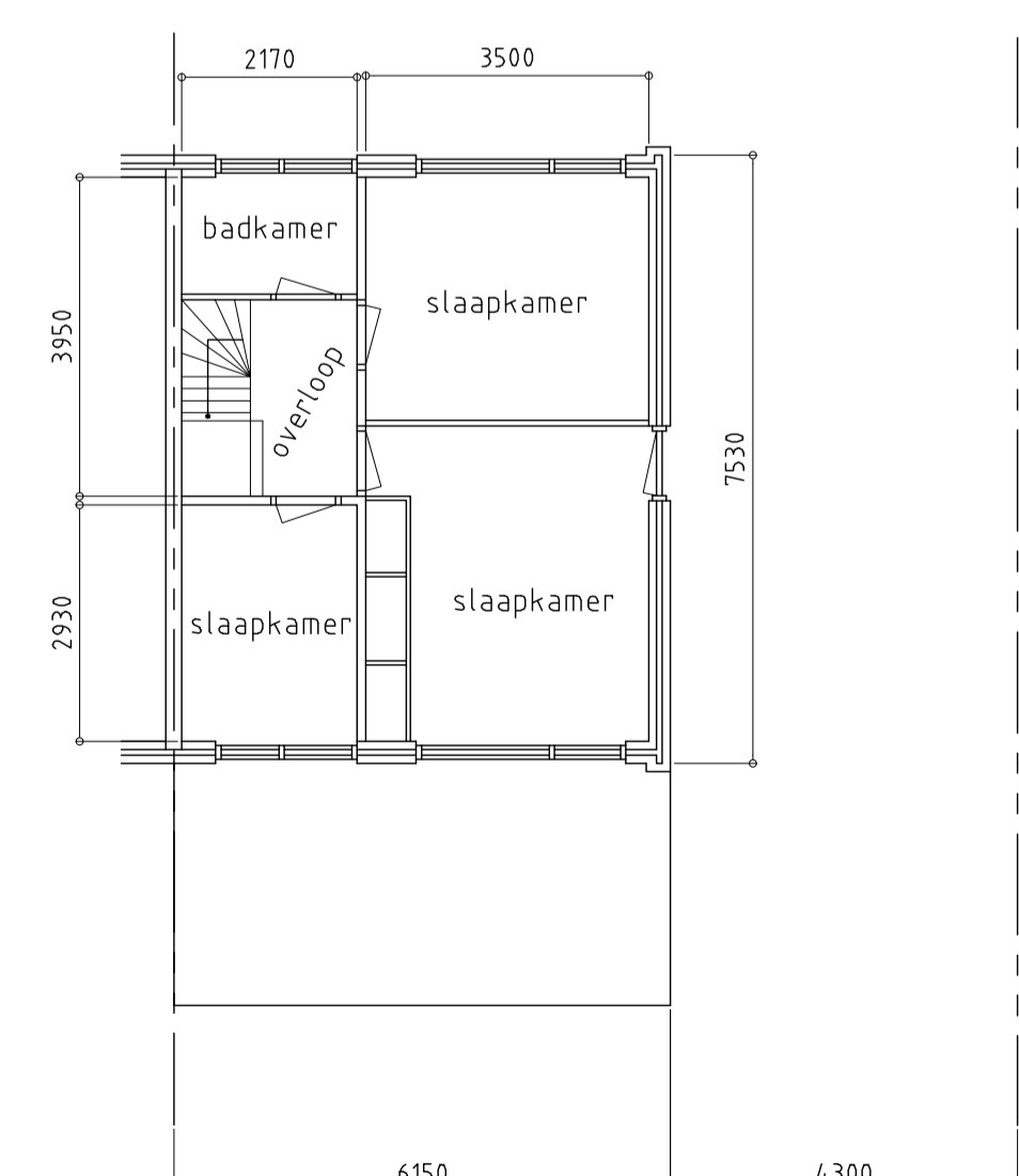
1e VERDIEPING BESTAAND
